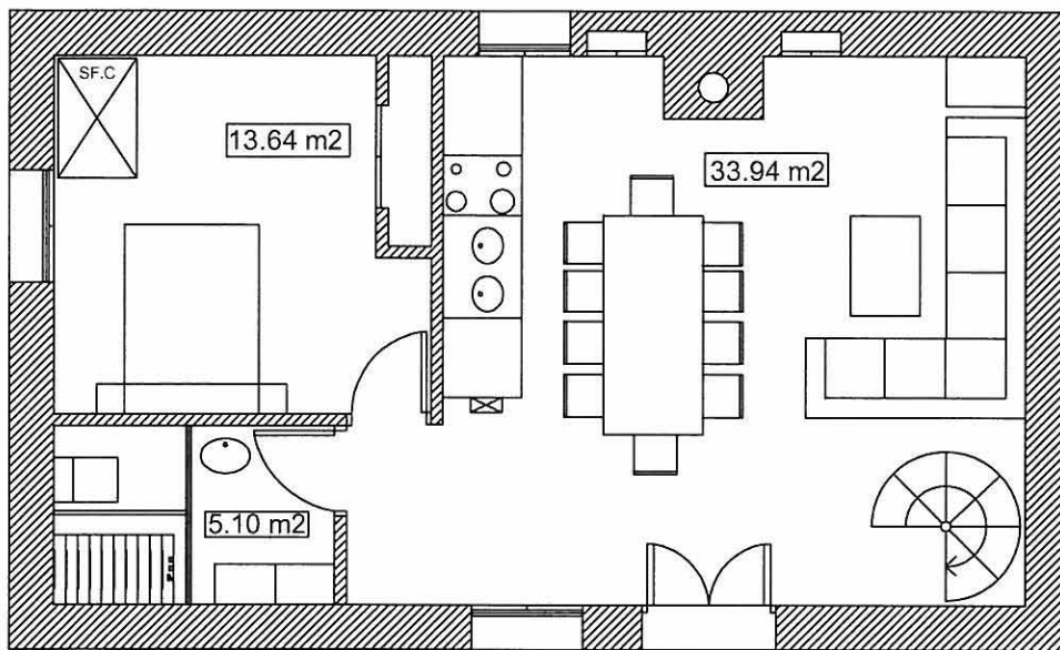
PLANTA BAJA
