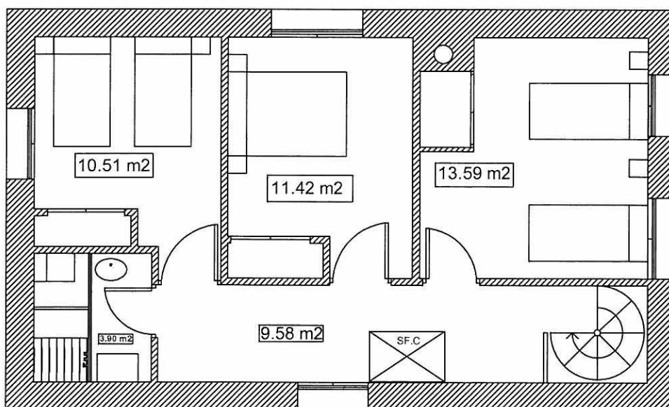
PLANTA 1º
