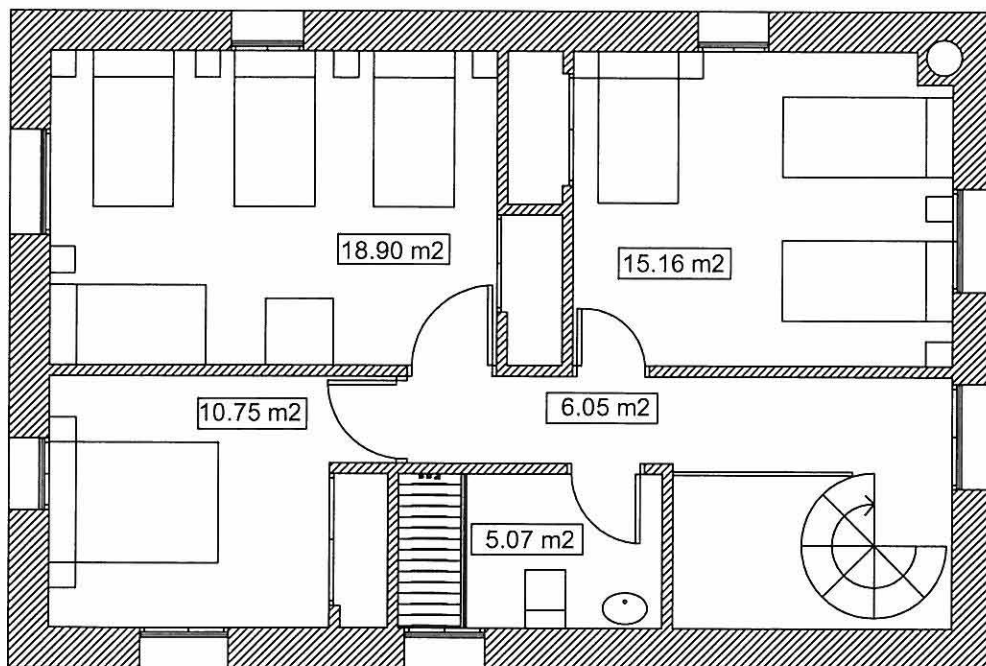
PLANTA ALTA
